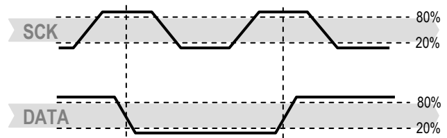
図 12：“Transmission Start”（通信開始）シーケンス
