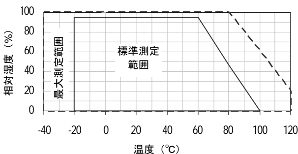
図 4：動作条件
